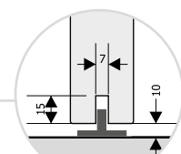
vodící trn
